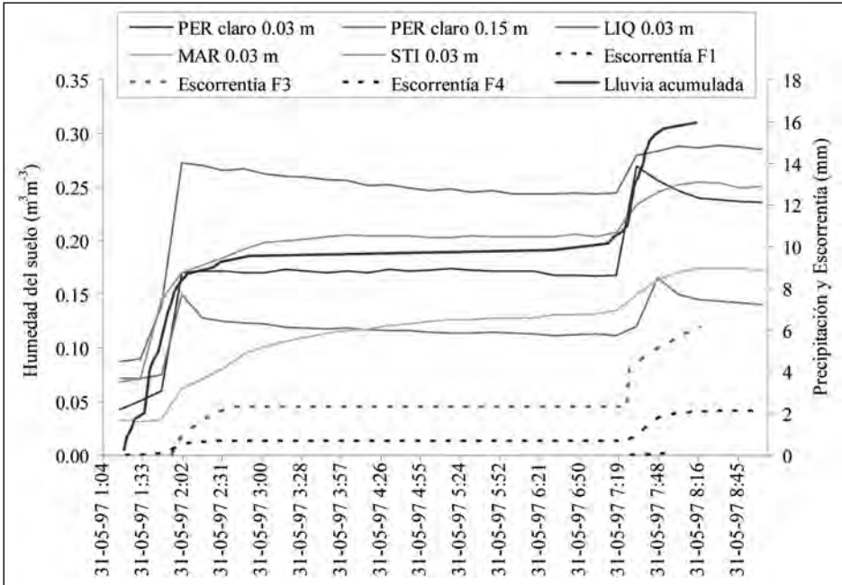
Figura 4. Evolución de la humedad del suelo a dos profundidades en cuatro diferentes geoformas durante dos eventos de precipitación en un mismo día y caudales generados en 3 afloradores. Permite ver que si el suelo está muy húmedo, unos pocos milímetros de lluvia son suficientes para generar de nuevo escorrentía. PER = pedimento cubierto de anuales y perennes; LIQ = ladera cubierta de líquenes; MAR = ladera desnuda; STI = ladera N cubierta de esparto
