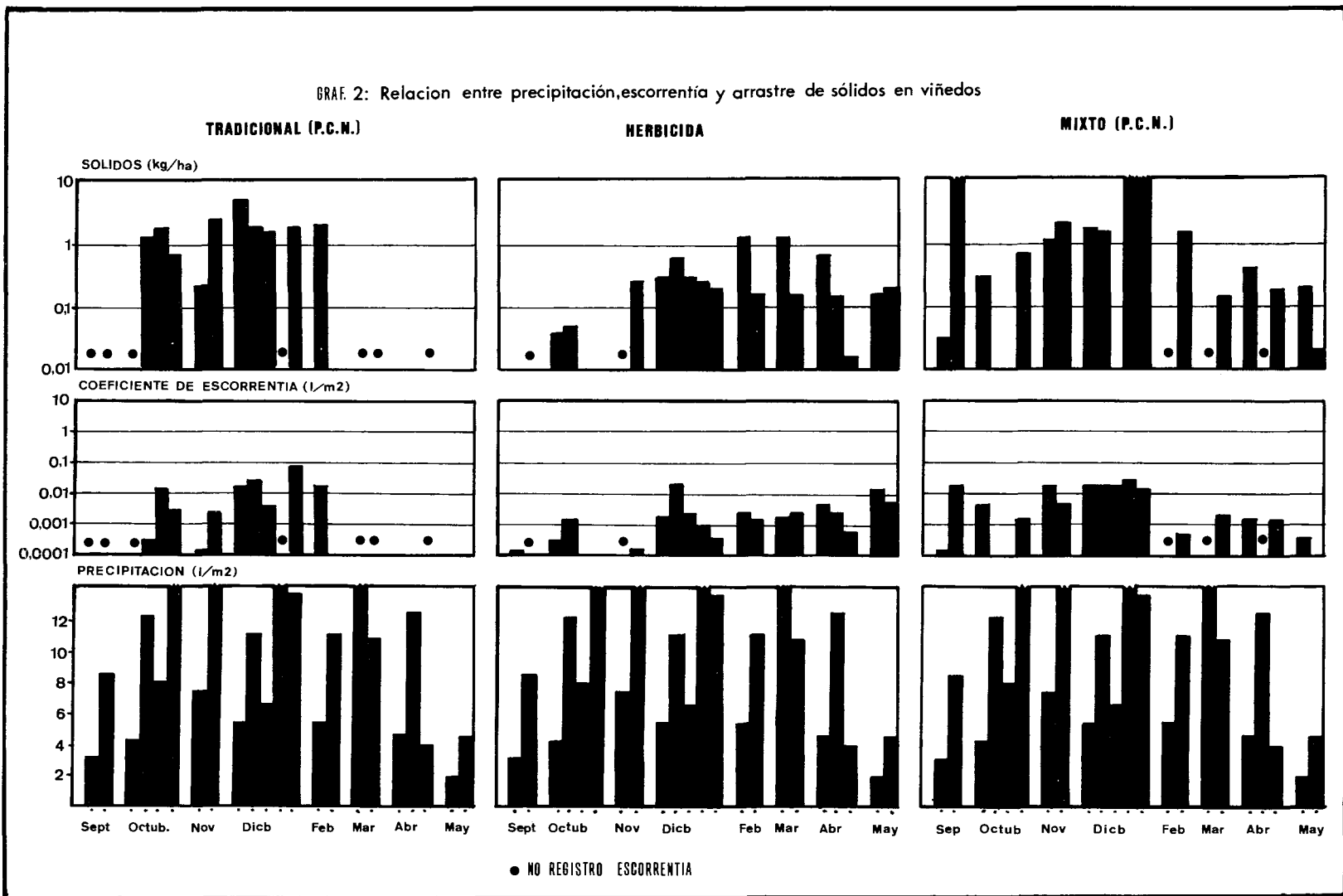
GRAF. N.º 2. RELACION ENTRE PRECIPITACIONES, ESCORRENTIA Y ARRASTRE DE SOLIDOS EN VIÑEDOS
